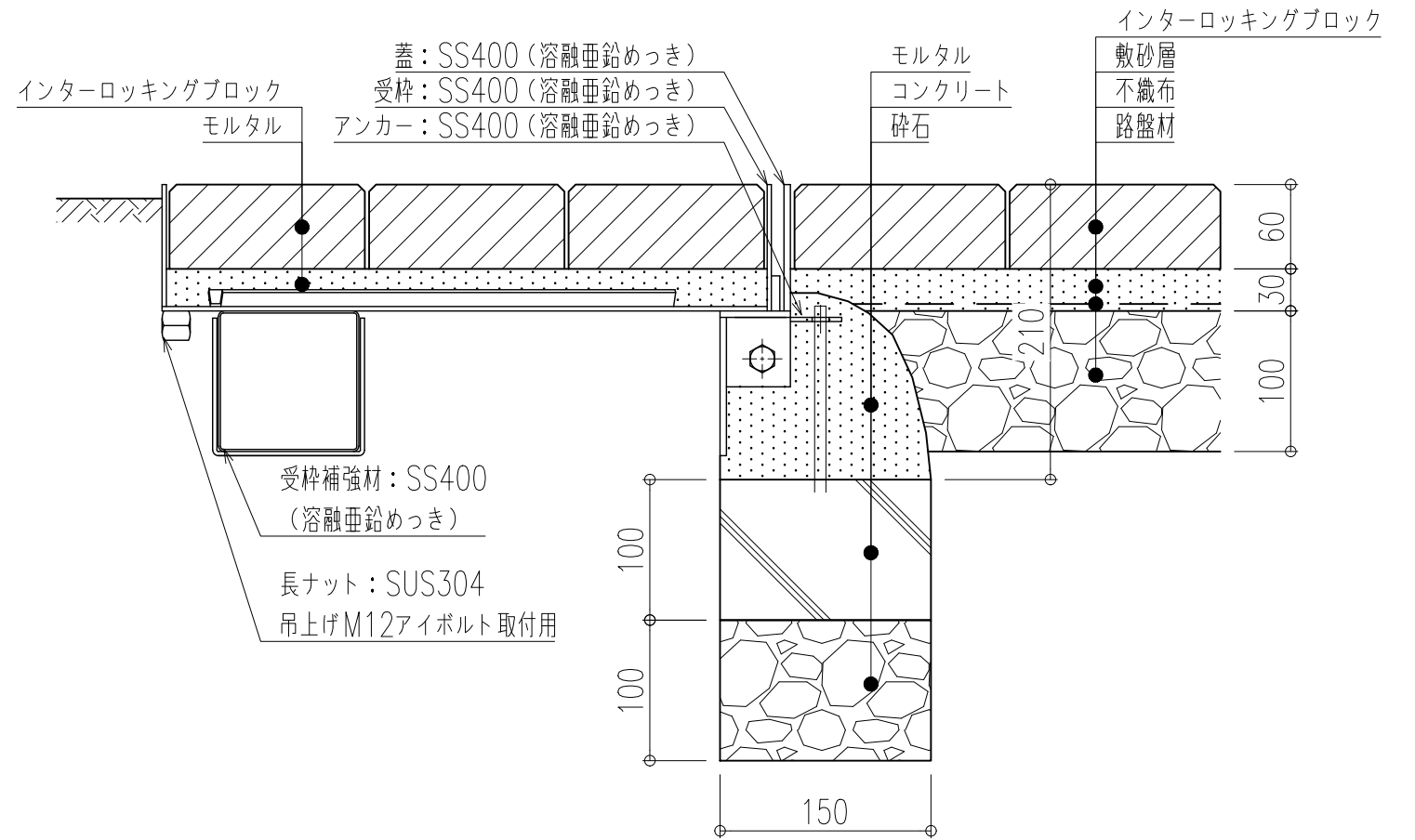
施工参考拡大図
