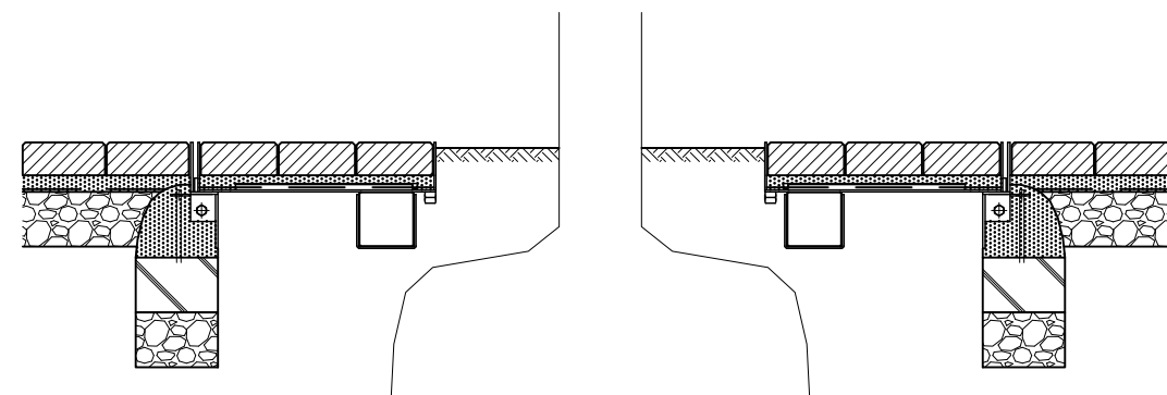
施工参考図
